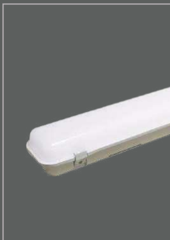
Zenda 12-52W 130Lm/W 4000K IP65 Optioneel met EPS
